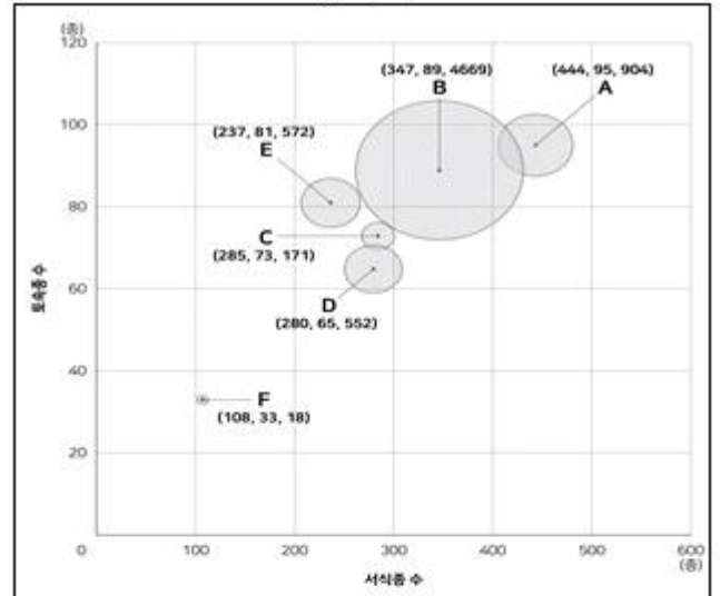
<그림> 갈라파고스 군도 A~F섬의 서식종 수, 토속종 수, 면적
