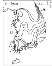
(가) 개나리 개화 시기
