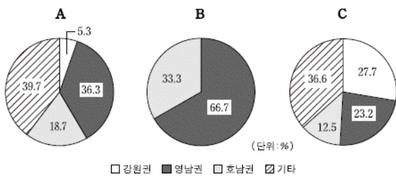
<1차 에너지 자원의 지역별 소비량 비중, 2007>
