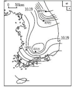
(나) 단풍 시작 시기
