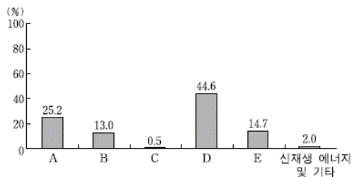
<우리나라의 1차 에너지 자원별 소비량 비중, 2007>
