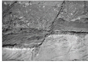
(나) 정단층
