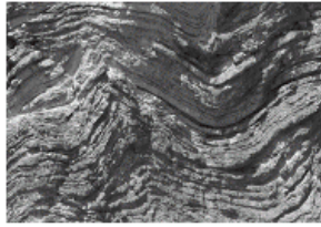
(가) 습곡
