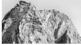
(나) 백령도 규암
