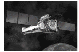
(나) 찬드라 X선 우주 망원경
